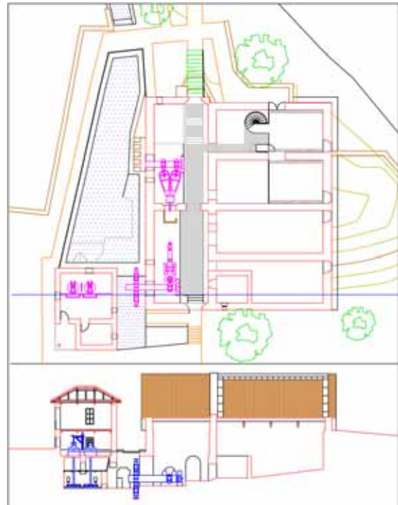
Planta de ferrería y molino
