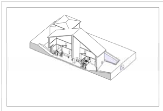
Perspectiva seccionada por salas de trabajo
